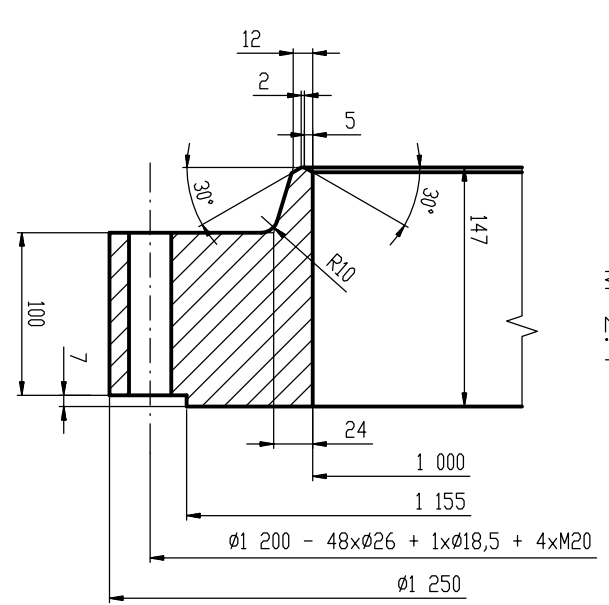
DETAIL B ДЕТАЛЬ Б М 2:1
