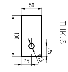
POS.18 ПОС.18 М 1:1
