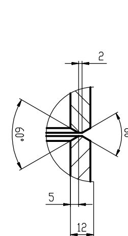
DETAIL I ДЕТАЛЬ И М 2:1
