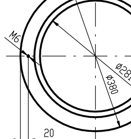
POS.7 ПОС.7 М 1:1
