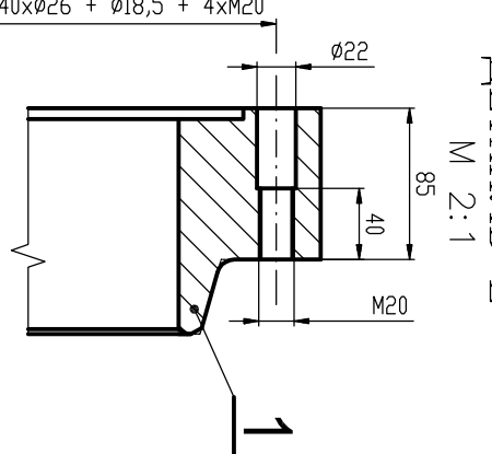
DETAIL E ДЕТАЛЬ Е М 2:1
