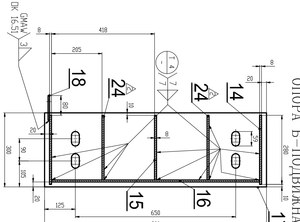
SLIDING SADDLE ОПОРА Б-ПОДВИЖНАЯ
