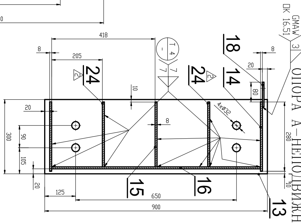
FIXED SADDLE ОПОРА А-НЕПОДВИЖНАЯ
