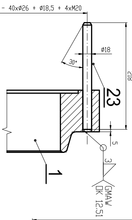
DETAIL C ДЕТАЛЬ Ц М 2:1
